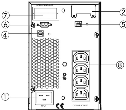
α. 1kVAS (DC24V) πίσω πίνακας
