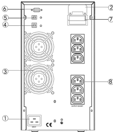
γ. 3kVAS (DC72V) πίσω πίνακας
