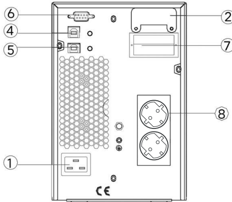
α. 1kVAS (DC24V) πίσω όψη
