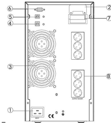
γ. 3kVAS (DC72V) πίσω όψη
