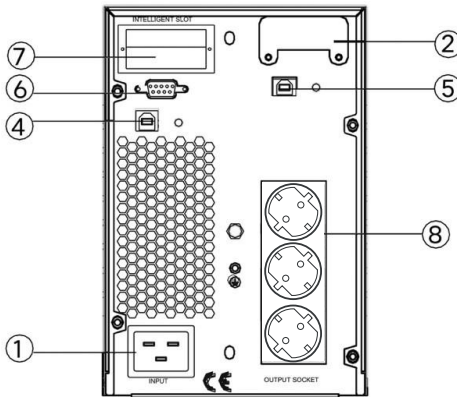
β. 2kVAS (DC48V) πίσω όψη
